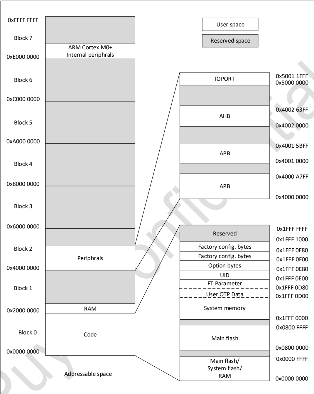
图 3-10 存储器映射
