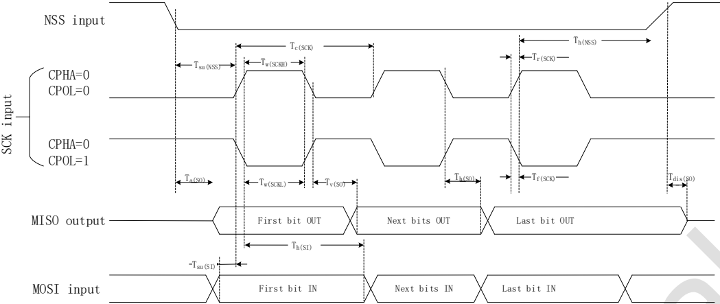
图 5-3 SPI 时序图-slave mode 和 CPHA=0
