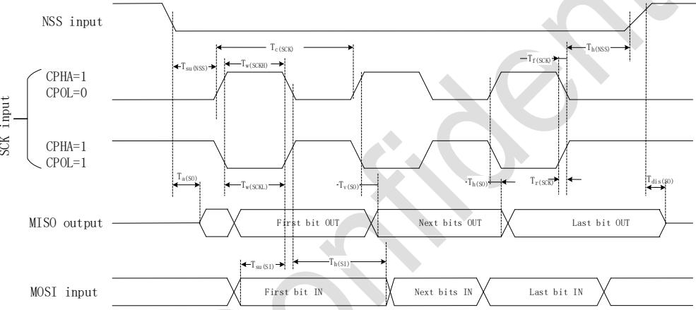
图 5-4 SPI 时序图-slave mode 和 CPHA=1
