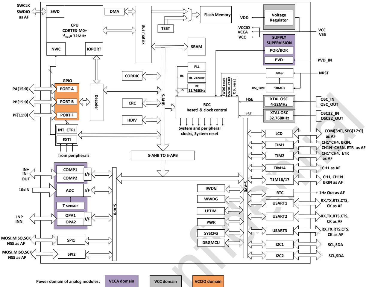
图 1-1 功能模块
