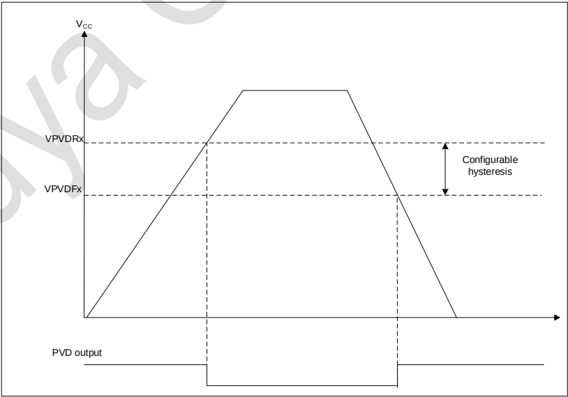
图 2-4 PVD 阈值
