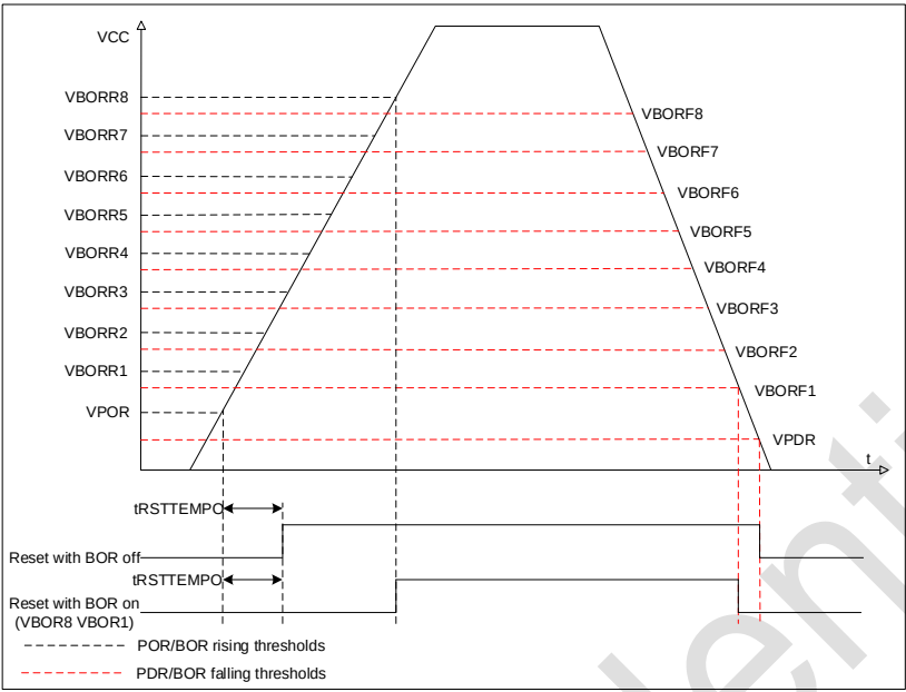
图 2-3 POR/PDR/BOR 阈值
