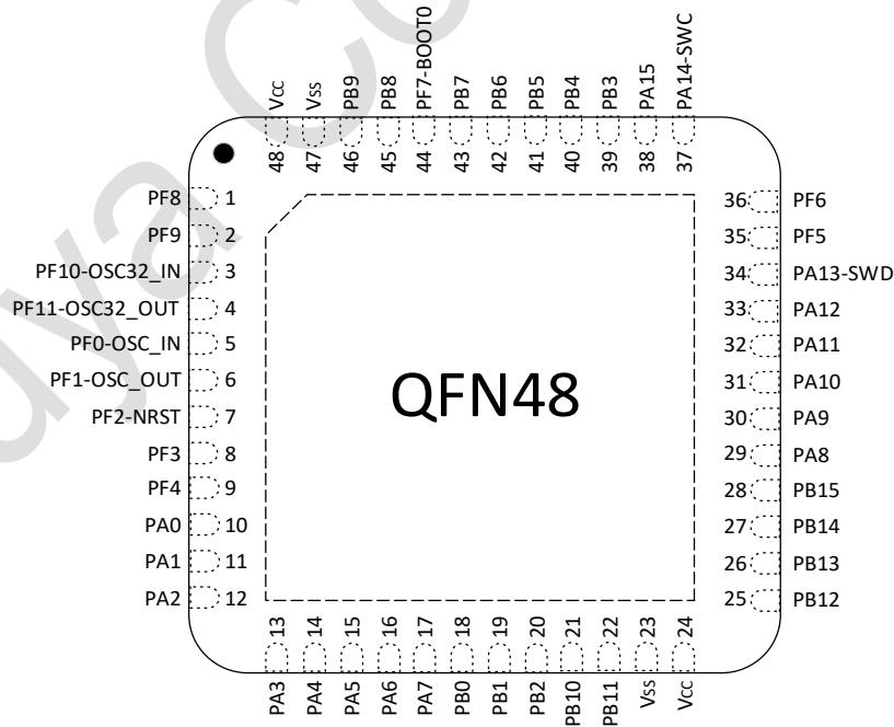
图 3-2 QFN48(6*6) Pinout1 PY32F031C1xU6 (Top view)
